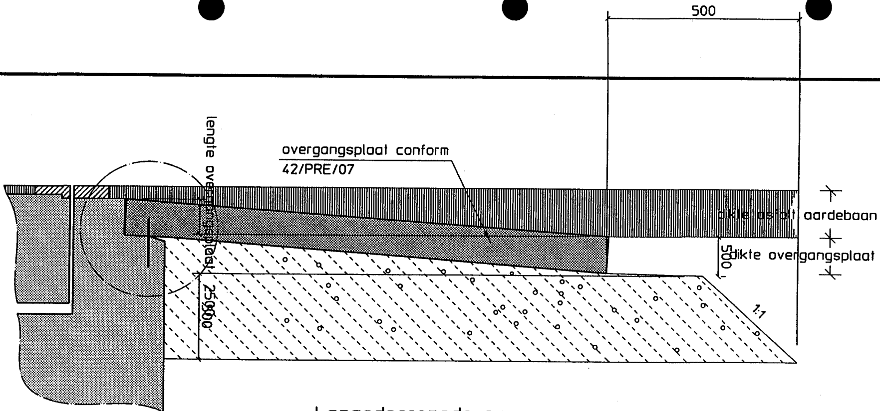
Langsdoorsnede Schaal 1:20
