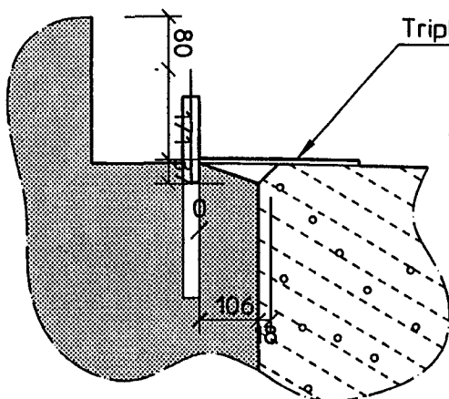
Detail oplegging overgangsplaat Schaal 1:10
