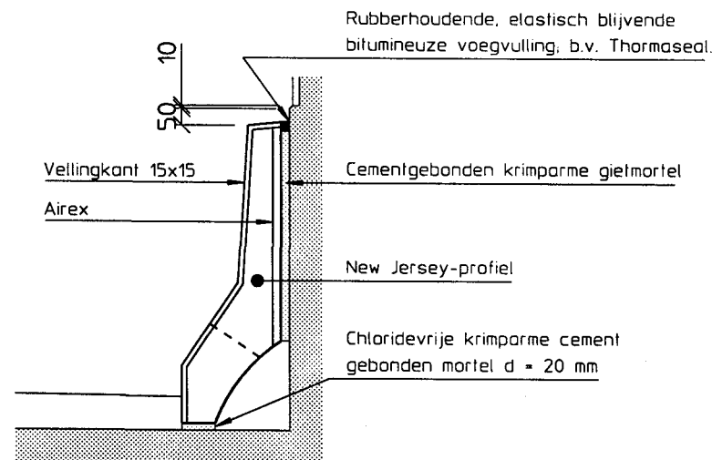
Doorsnede t.p.v. voeg
