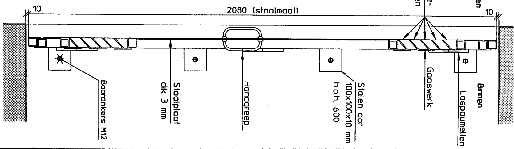
Doorsnede B-B 1:10
