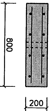
Dwarsdoorsnede
