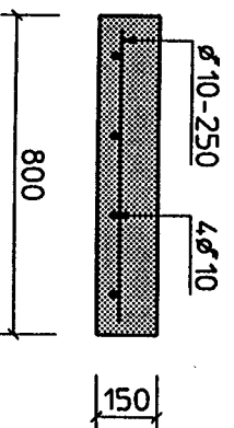
Langsdoorsnede
