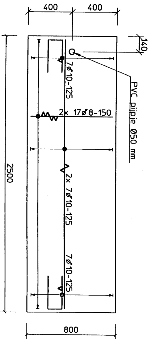
Bovenaanzicht
