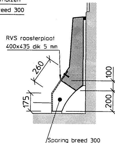
Doorsnede A
