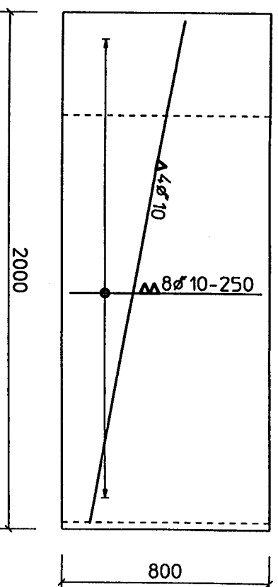
Bovenaanzicht
