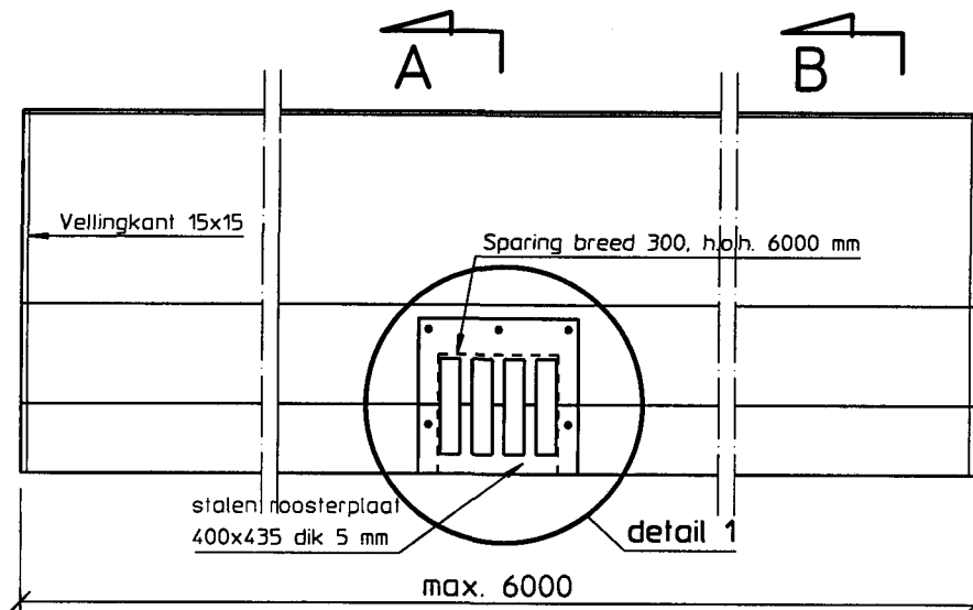
Aanzicht New-Jersey
